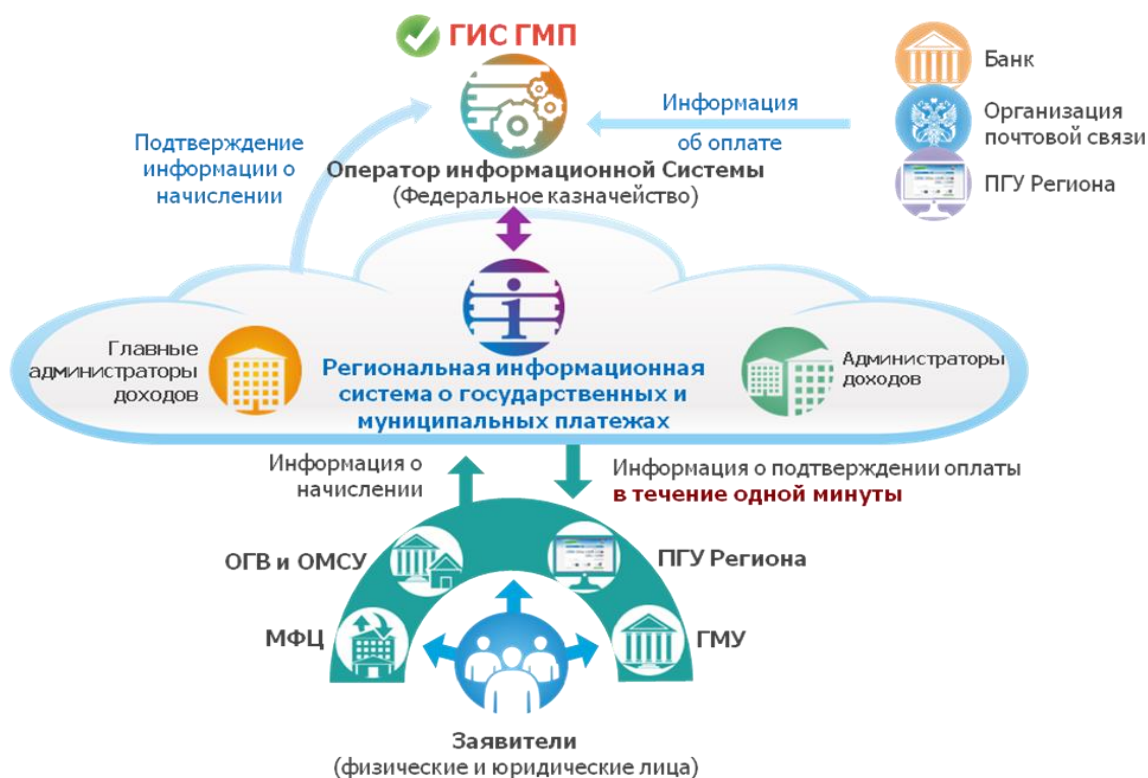
Рис. 2 – схема взаимодействия с федеральным сервисом ГИС ГМП
